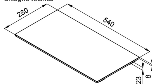
Disegno tecnico
