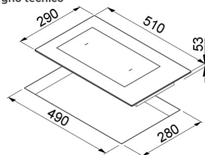
Disegno tecnico
