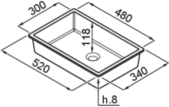
Disegno tecnico
