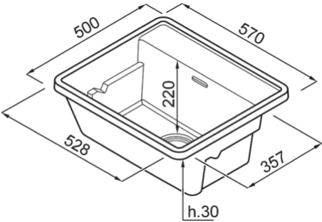
Disegno tecnico
