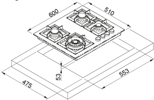
Disegno tecnico
