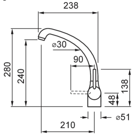
Disegno tecnico
